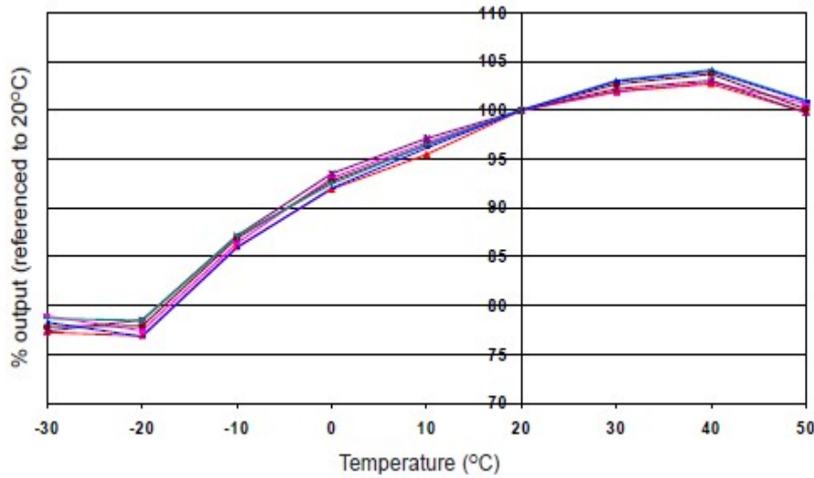
图1 灵敏度温度特性
