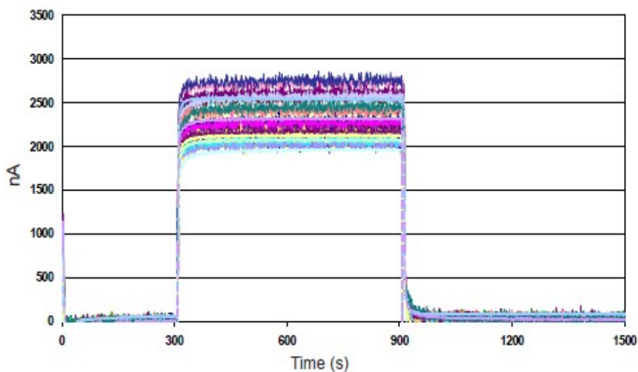
图3 对10ppm SO 2 的反应
